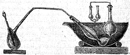
Фиг. 1. Приборъ для опредѣленія іода въ іодистыхъ металлахъ и пр.
