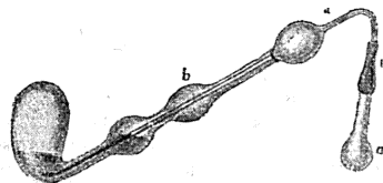
Фиг. 2. Приборъ для опредѣленія хлора, перекисей и пр.
