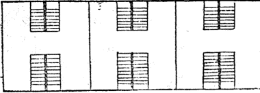
Фиг. 2. Вобановскія казармы уже безъ продольной капитальной стѣны.
