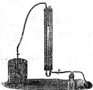
Фиг. 4. Приборъ для опредѣленія кислотъ иодометрическимъ способомъ по выдѣленію кислорода изъ перекиси водорода.
