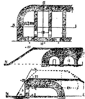
Фиг. II (профиль).
