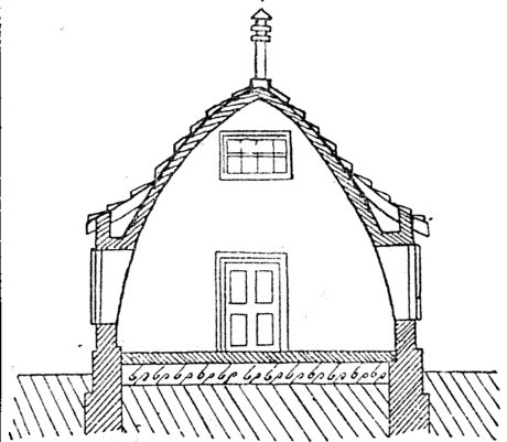
Фиг. 4. Казарма стрѣлчатой системы Толле.
